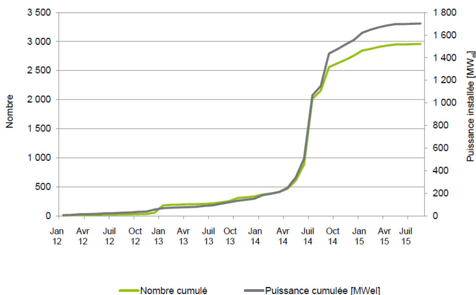
Figure 4-1 : Cumul du nombre d'installations inscrites au dispositif d'accès à la prime de flexibilité et de leur puissance électrique installée (Scheftelowitz et al., 2015)
